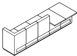
5 W4000 D875/1175 H750/900/1100 mm
