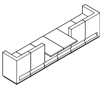
6 W4800 D875/1175 H750/900/1100 mm
