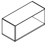
AS07 Open Top W900 D380 H400 mm
