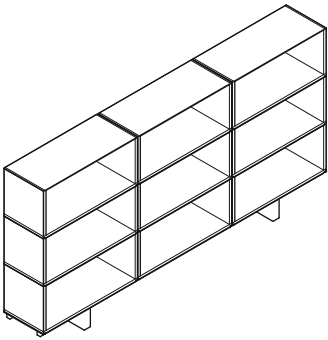
4 W2700 D380 H1370 mm
