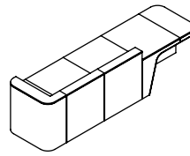
3 W3200 D875 H750/900/1100 mm
